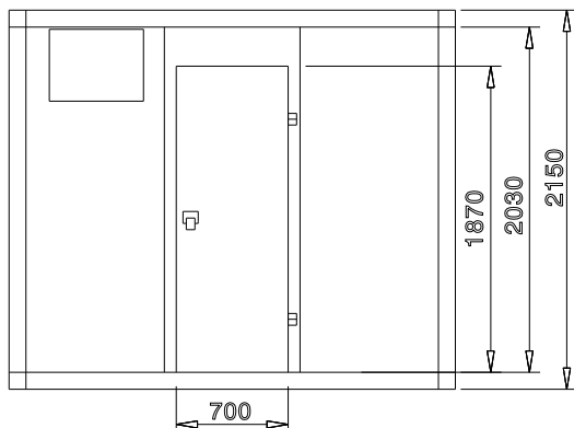
Boční
